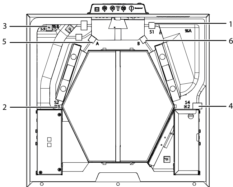
Fig. 12: Positionnement des sondes
