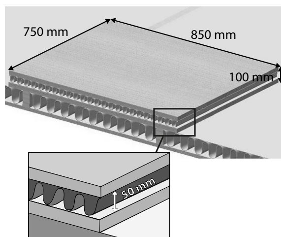
Fig. 43: Fabrication d'une structure porteuse en bois
