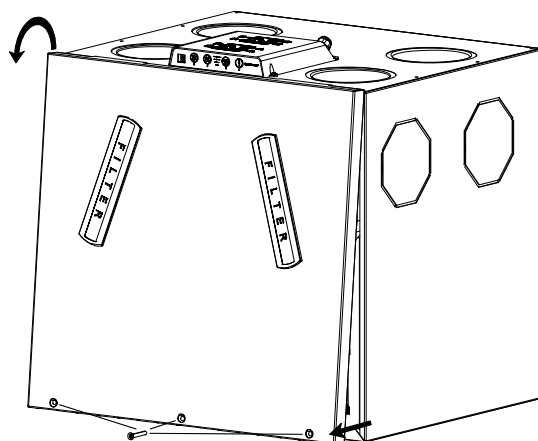
Fig. 32: Dépose de la face avant
