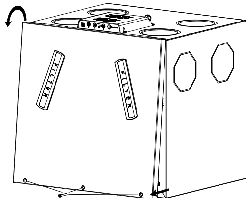
Fig. 57: Dépose de la face avant
