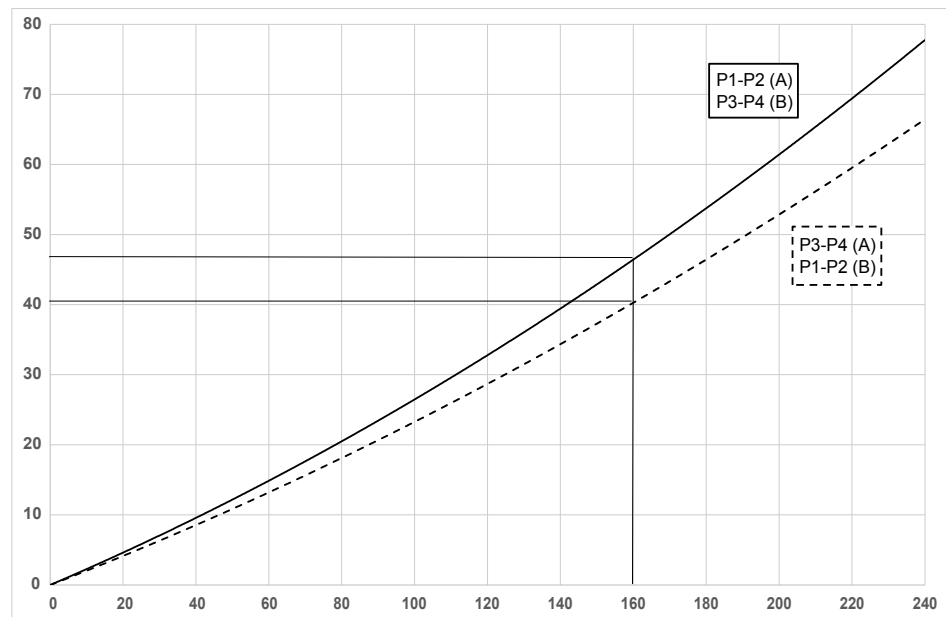
Fig. 54: Graphique de débit
