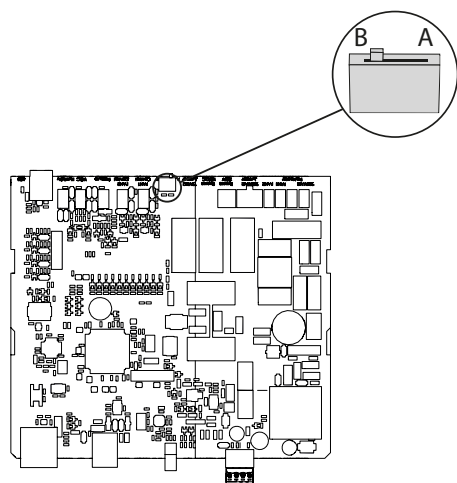
Fig. 45: Vérification du mode de fonctionnement
