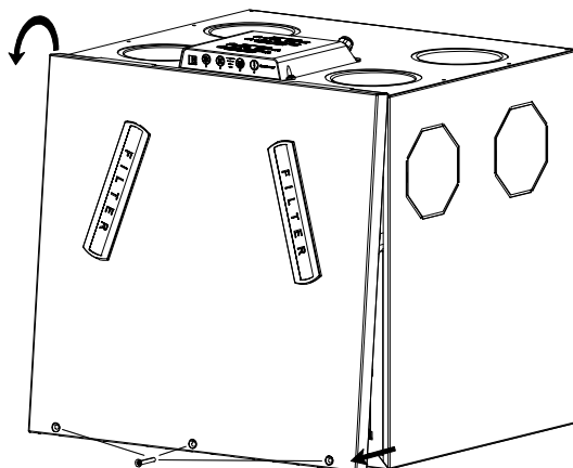
Fig. 28: Dépose de la face avant
