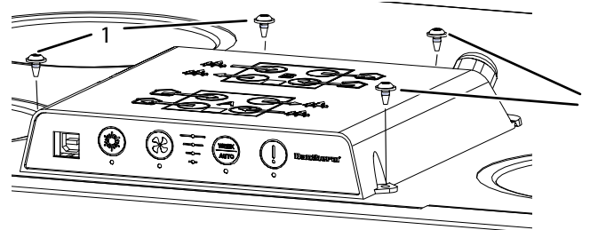
Fig. 26: Dévisser les vis
