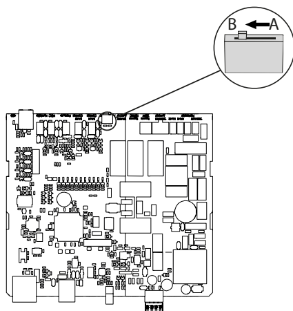
Fig. 31: Passage du commutateur sur Mode B.
